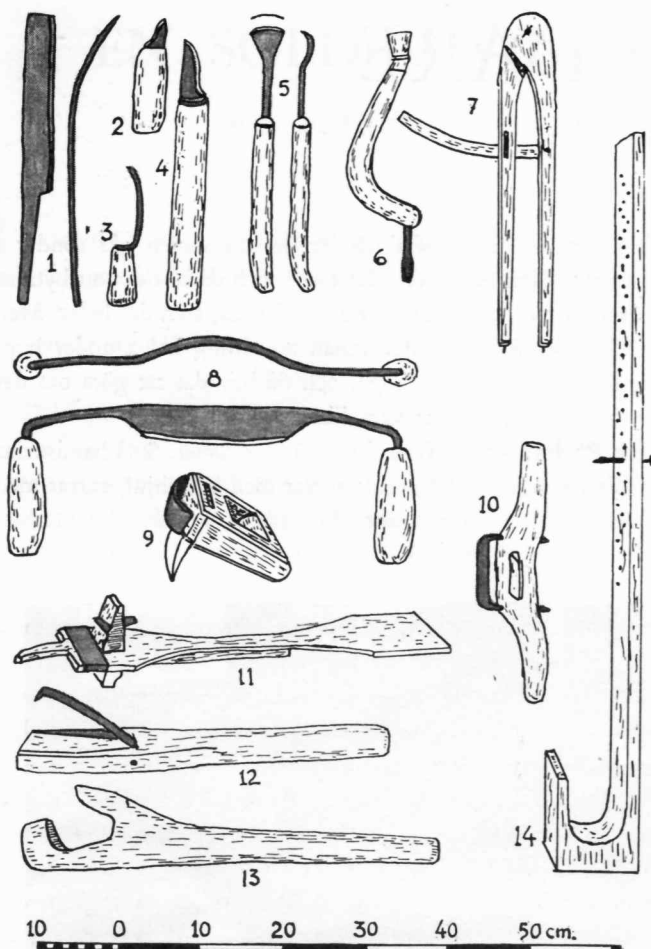
Redskap för laggkärlstillverkning: 1. Skavjärn; 2. Ristjärn; 3. Skjutjärn; 4. Bandkniv; 5. Skjutjärn; 6. Dymlingborr; 7. Passare; 8. Laggkniv; 9. Innerskave; 10. Ytterskave; 11. Laggsåg; 12. Bandhake; 13. Bandhake; 14. Ritmått;
