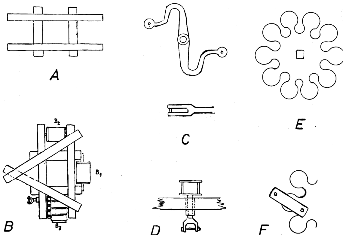
2. A. Ramkonstruktion. B. Maskinen, sedd uppi från. C. Den dubbelt S-formade armen, i vilken de vridbara klorna är fästade. D. Kuggdrivaren. E. Kugghjulet. F. Kuggdrivarens verkningssätt.
