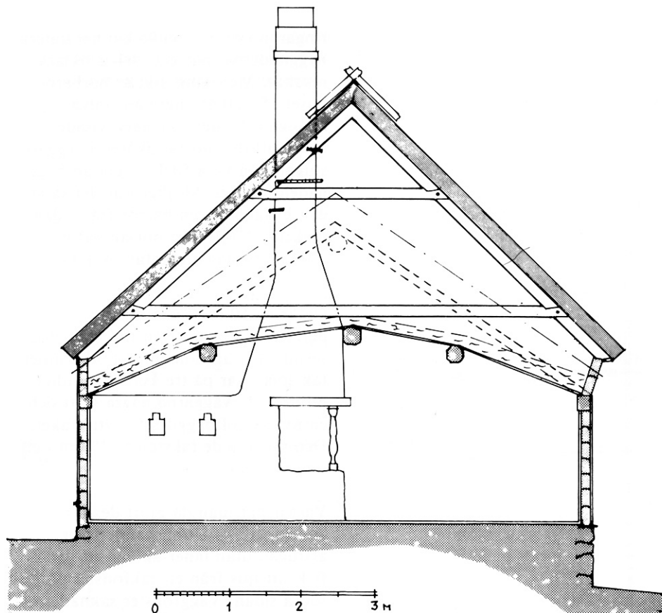
Sektion av "stugan". Ritningen visar hur takkonstruktionen successivt förändrats. Uppmätning och ritning av Christer Råsbäck 1985.
