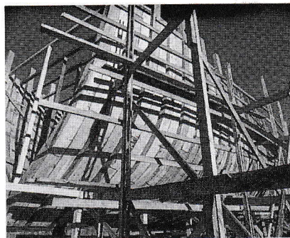
54 SPANT skall resas innan bordlägg- ningen kan ske. Det tyngsta spantet väger ca 1,5 ton. Höjden på spanten är ca 5,6 m. Bredd 48 cm.
