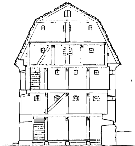
SEKTION (UPPMÄTN. NORD. HÅLLET)
