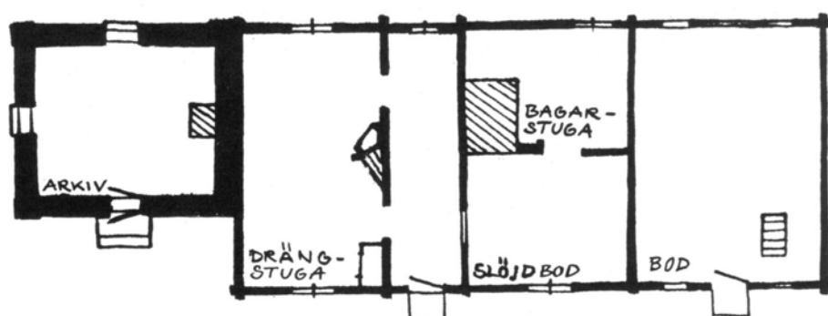
Planritning av den södra flygelbyggnadens bottenvåning efter 1916 års tillbyggnad av ett arkiv mot öster.
