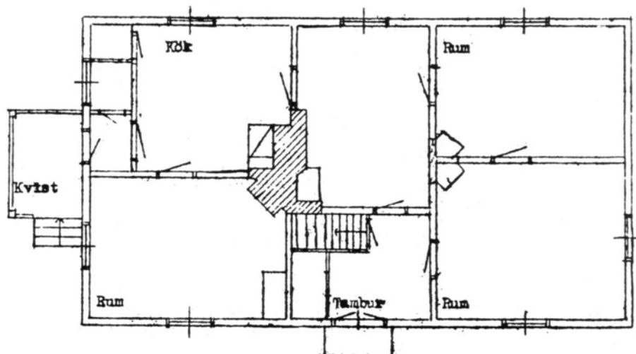
Uppmätning av den norra flygelbyggnaden den 31.1 1949. R.K.
