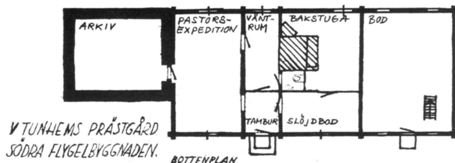
Planritning av den södra flygelbyggnadens bottenvåning efter 1916 års tillbyggnad av ett arkiv mot öster.
